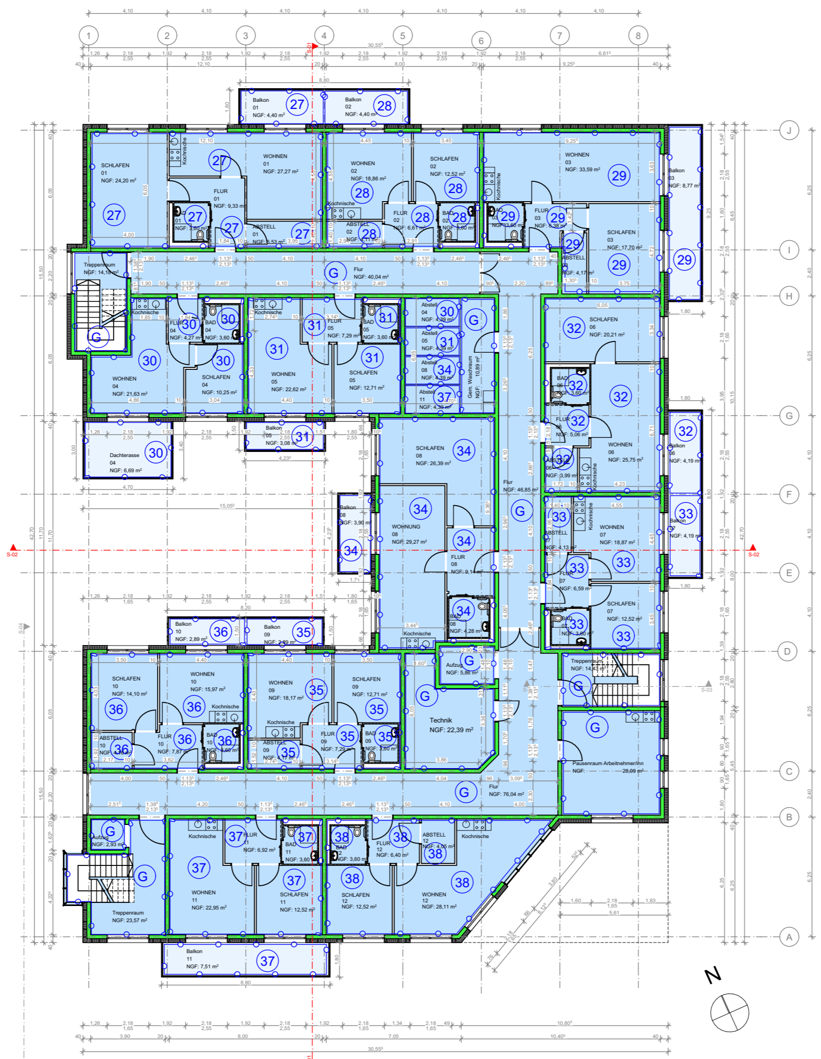
2. OBERGESCHOSS BGF: 1086 MZ
