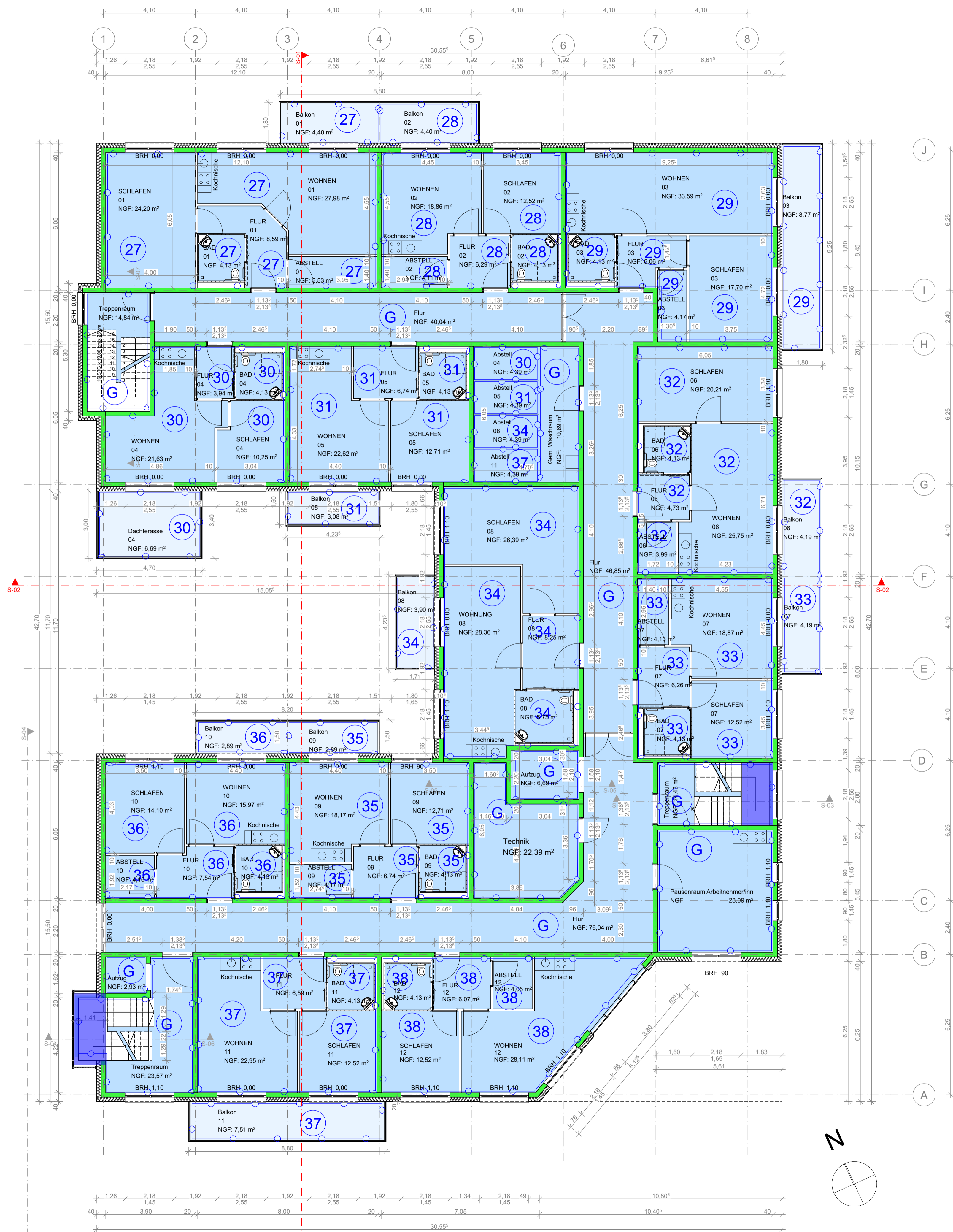
2. OBERGESCHOSS BGF: 1086 M 2
