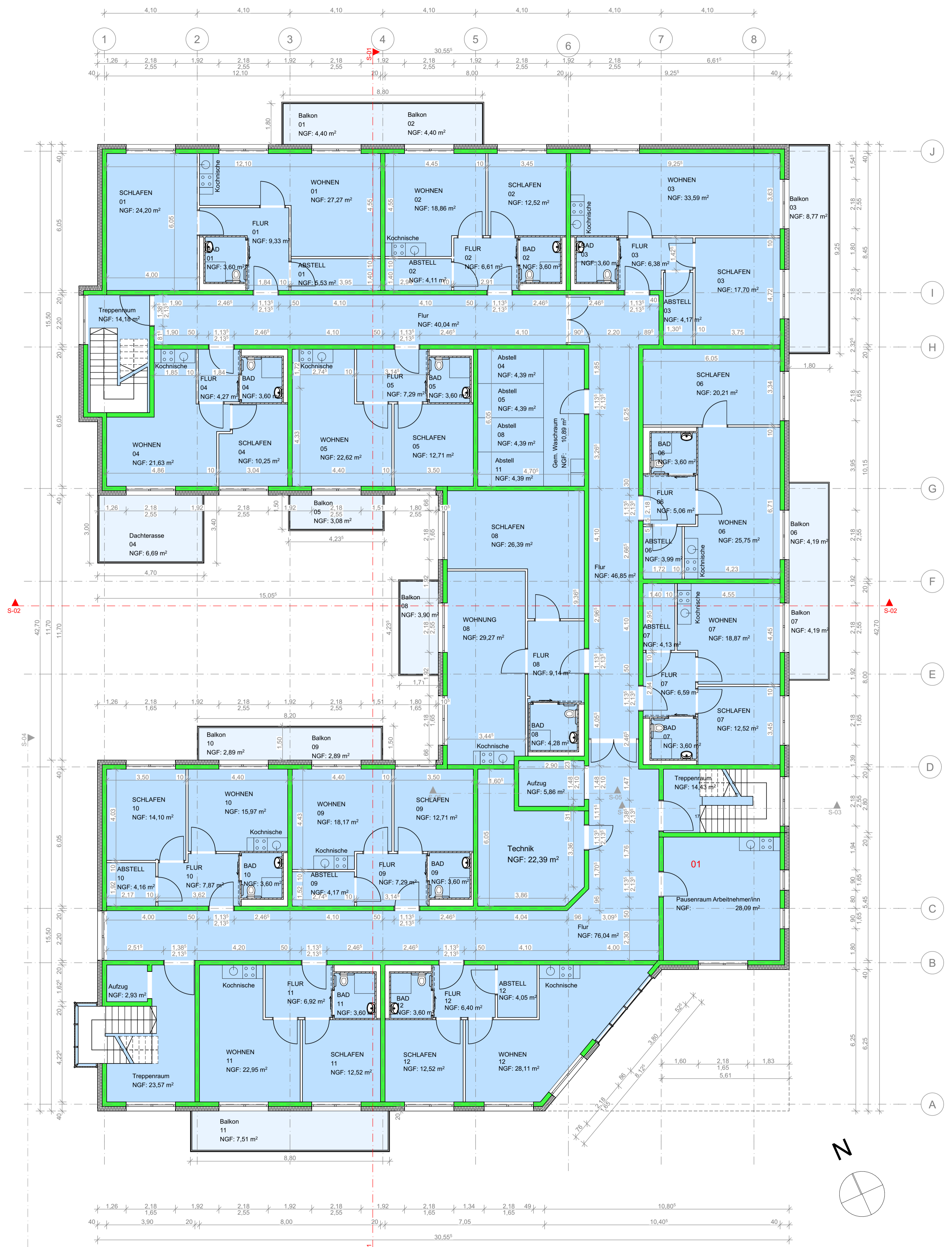
2. OBERGESCHOSS BGF: 1086 M 2
